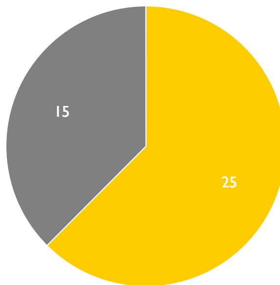
Rücklaufquote 62,50%
